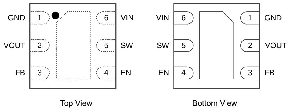
DFN6 (ET82099Y)
