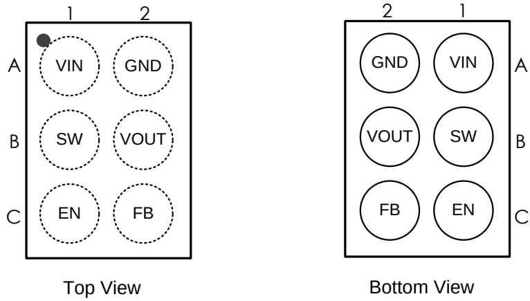
WLCSP6 (ET82099)
