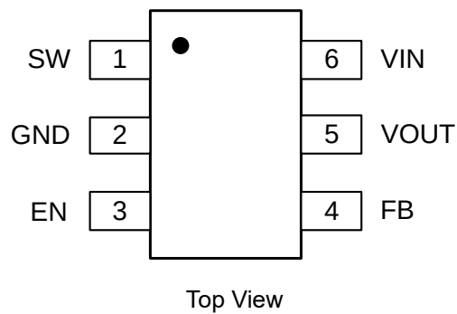
SOT23-6(ET82099S)
