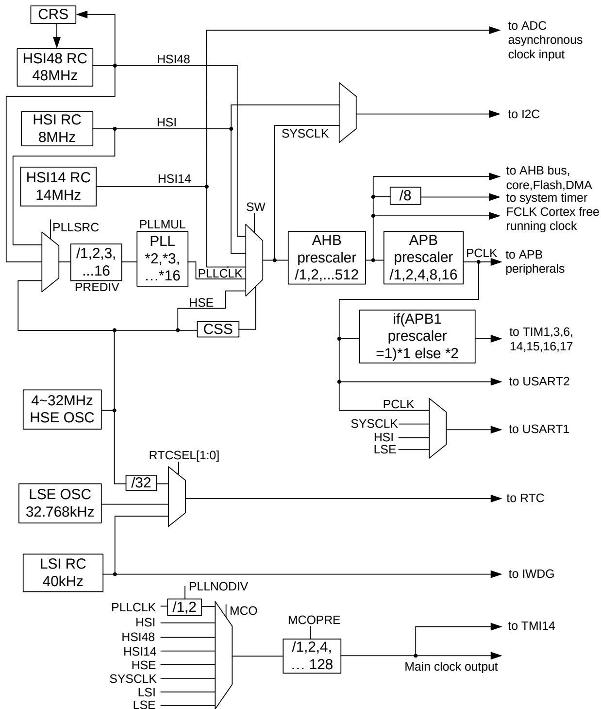
图 3.1 时钟框图
