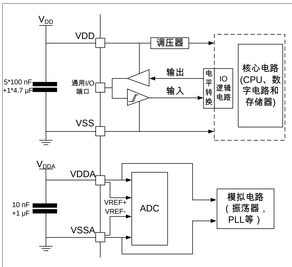
图 6.3 供电方案图
