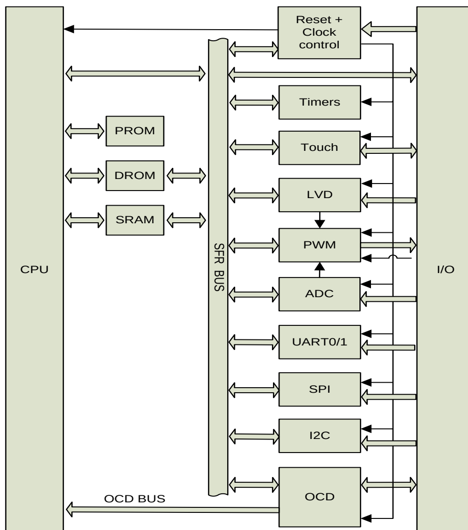
图 1-1 系统结构框图
