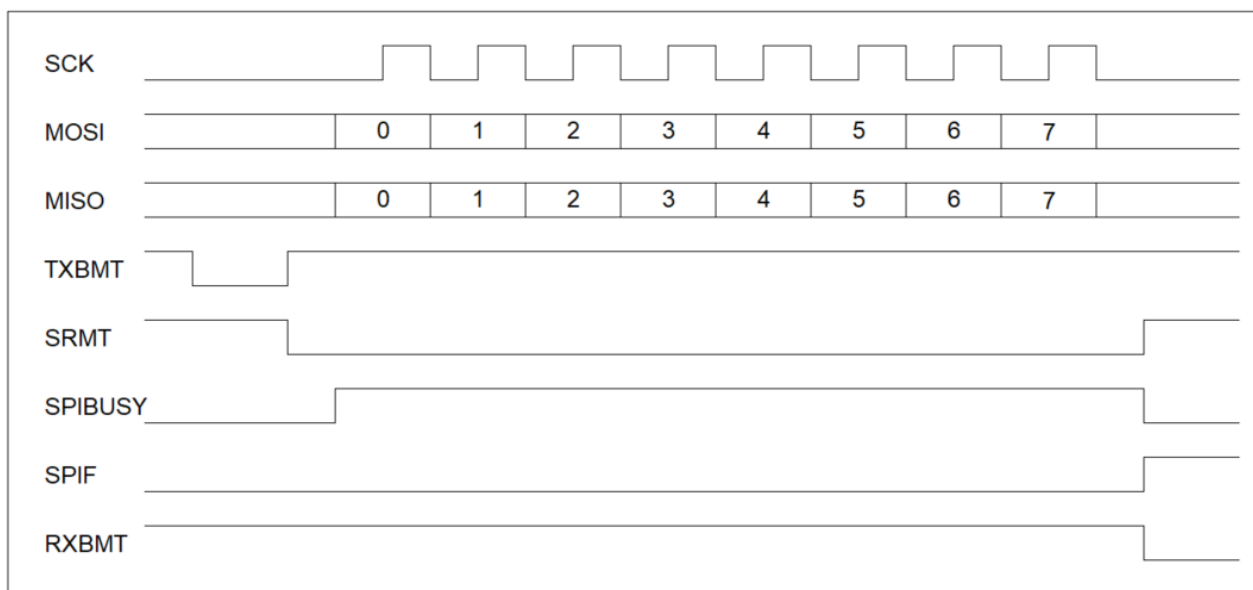
图 11-5 数据处理时序图 (以单字节数据传输为例)
