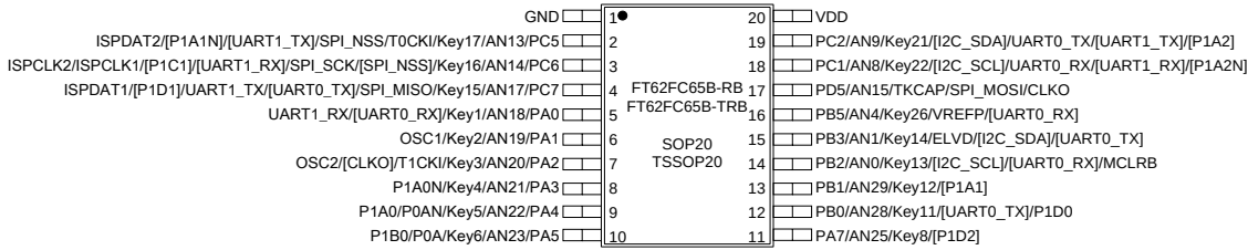
图 1-6 SOP20 / TSSOP20 (B) 1
