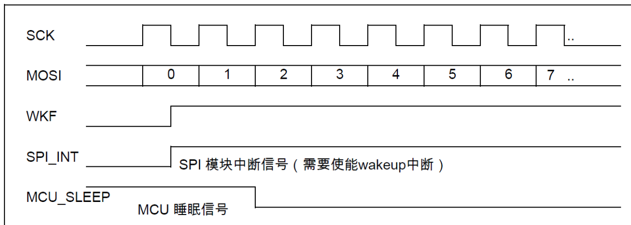
图 11-6 睡眠唤醒时序图
