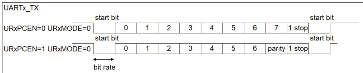
图 13-2 异步模式通信格式 (以 8bit 数据格式为例)
