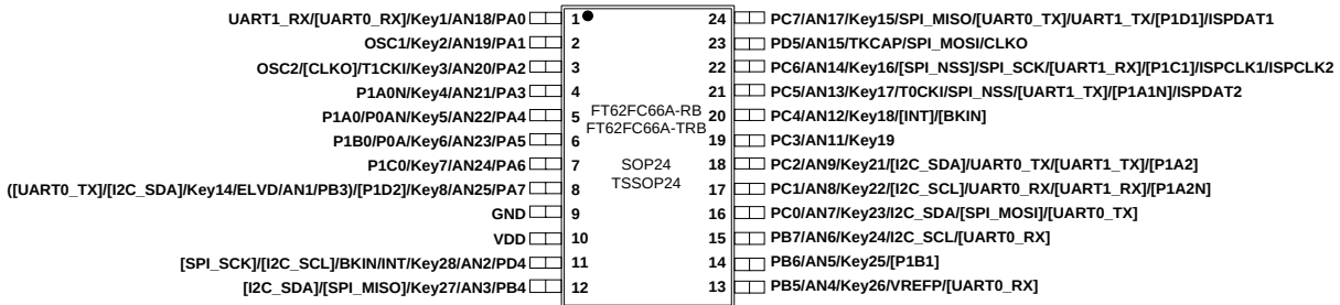
图 1-7 SOP24 / TSSOP24 (A) 1,2
