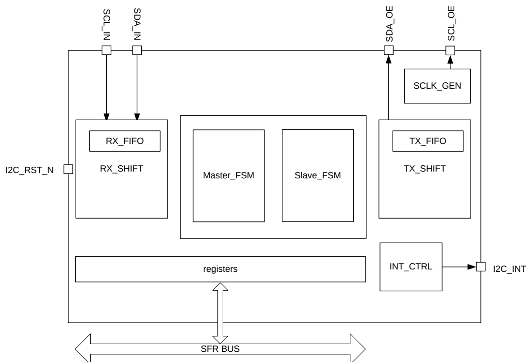
图 12-1 I2C 结构框图
