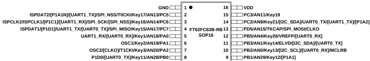
图 1-4 SOP16 (B) 1
