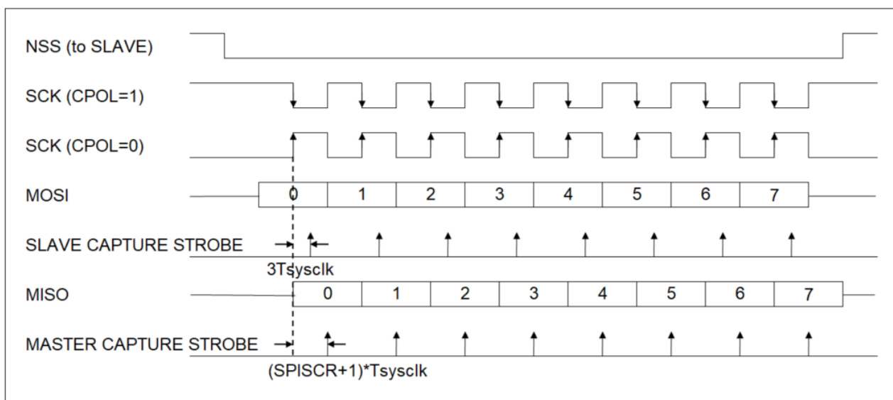
图 11-3 时钟极性 CPHA=0 时序图 (以 LSBFIRST = 1 为例)
