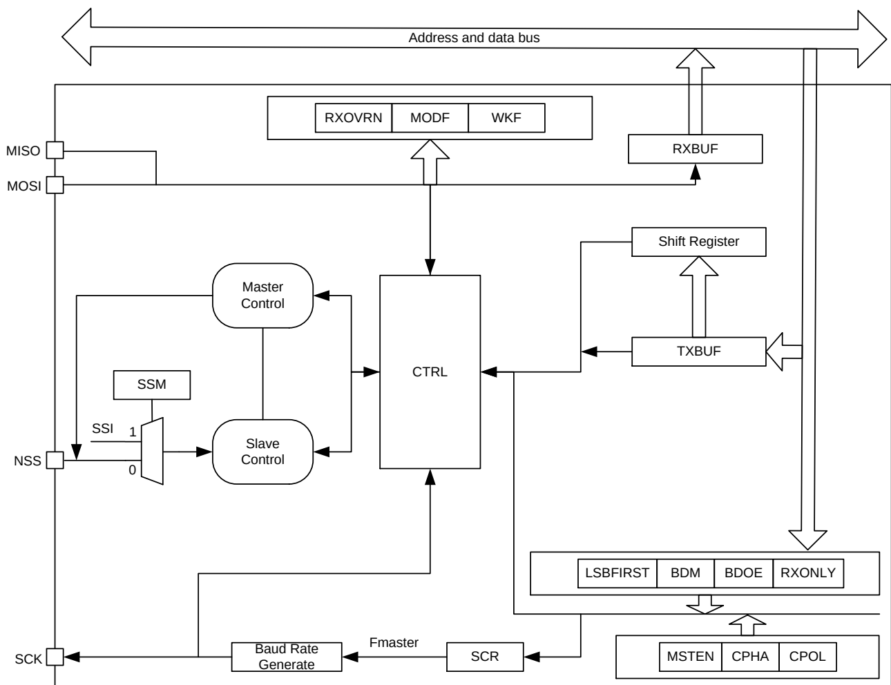
图 11-1 SPI 结构框图
