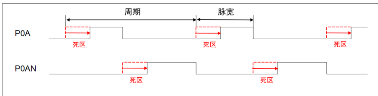
图 7-3 PWM0 时序图
