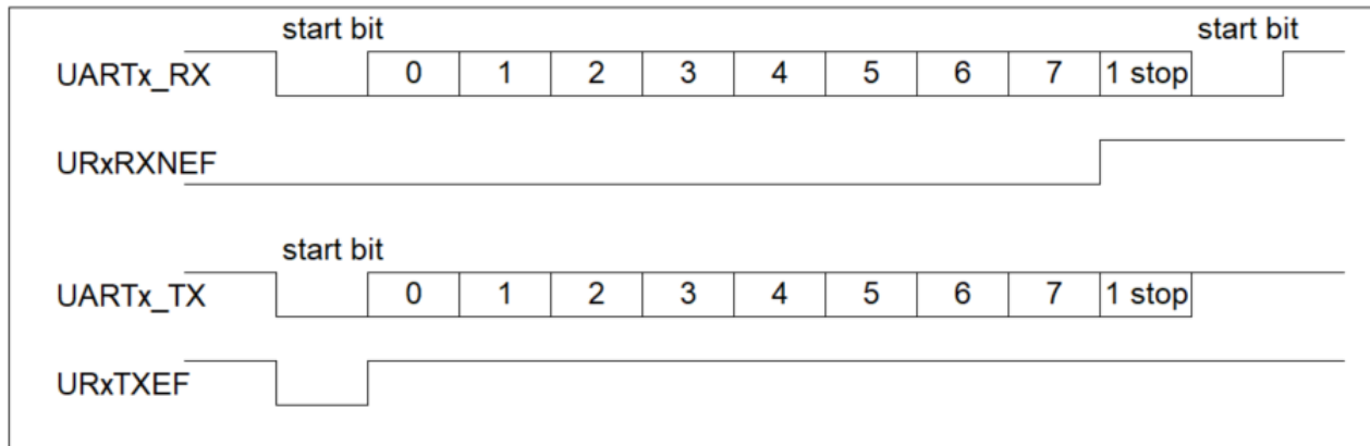
图 13-3 异步模式标志位时序图
