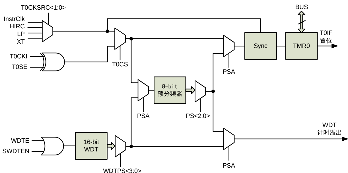
图 7-2 Timer0 结构框图
