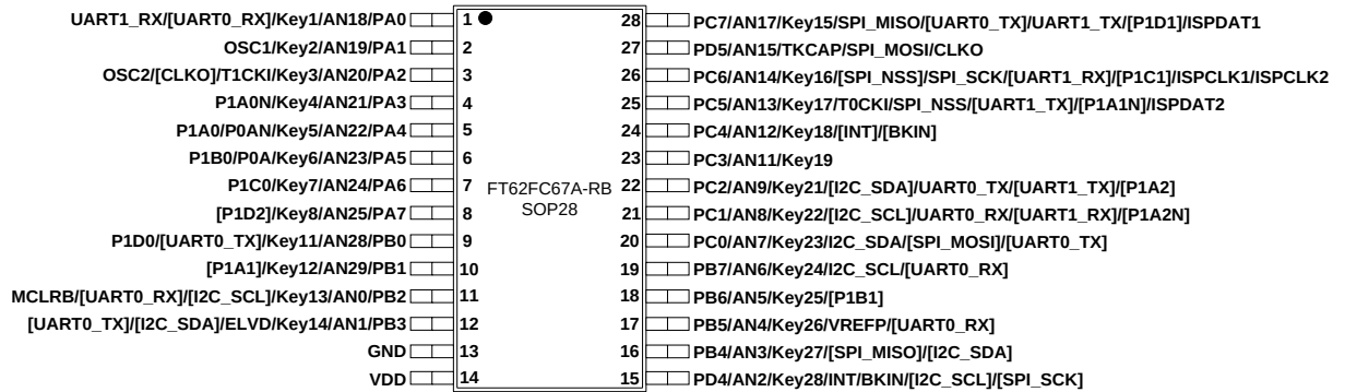
图 1-8 SOP28 (A) 1
