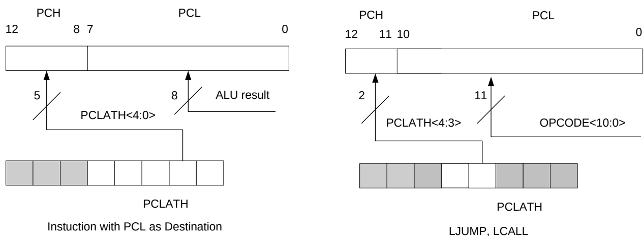
图 17-2 装载 PC 值的不同情况
