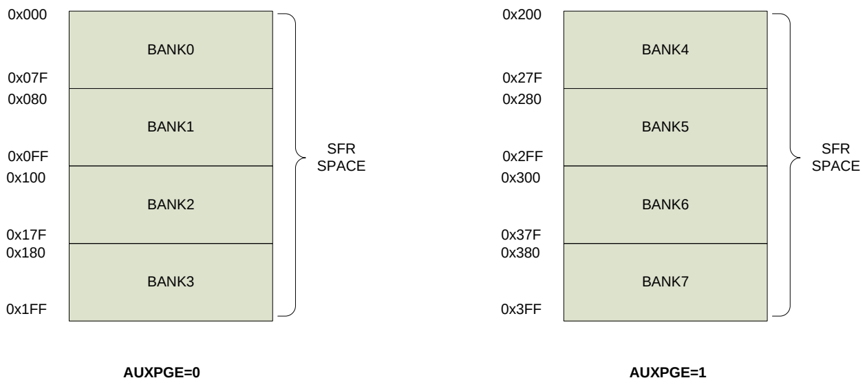
图 17-3 间接寻址
