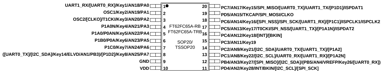
图 1-5 SOP20 / TSSOP20 (A) 1 2
