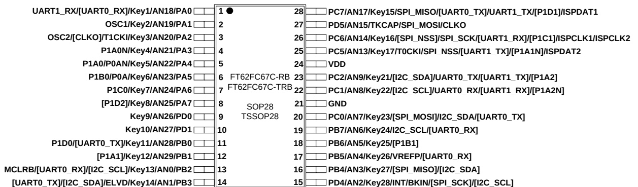
图 1-9 SOP28 / TSSOP28 (C) 1
