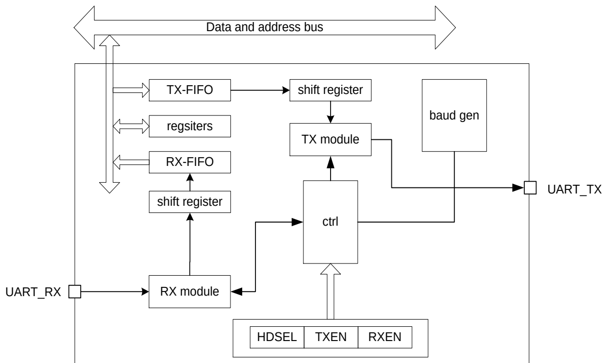
图 13-1 UART 结构框图
