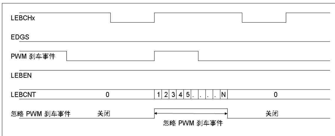
图 8-3 LEB 时序图
