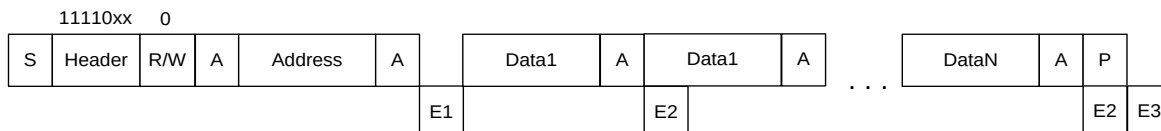
图 12-5 从机接收流程
