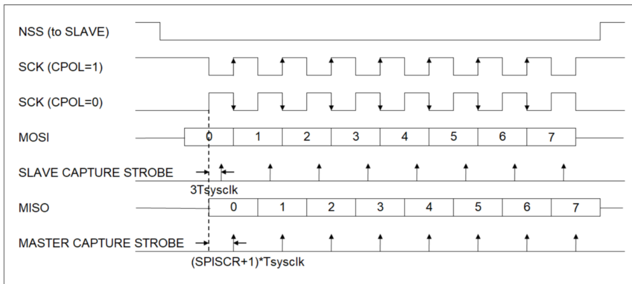
图 11-4 时钟极性 CPHA=1 时序图 (以 LSBFIRST = 1 为例)
